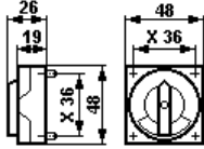
Ex 23 switch actuator
