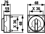
Tête de commutateur de commande Ex 23
