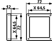
Messinstrumentvorsatz AM 72
