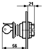
Schlagastervorsatz "NOT-AUS" mit Schlüsselentriegelung
