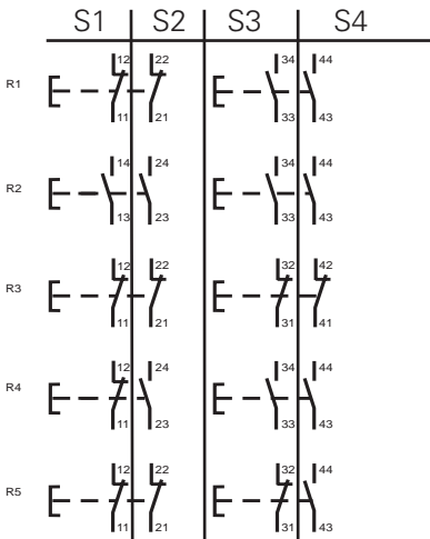
Schlagtaster mit verstärkter Verrastung GHG 410 1437R....
