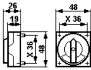
Schaltvorsatz für Ex 23
