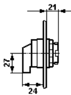
Tête de commutateur de commande et de potentiomètre *1
